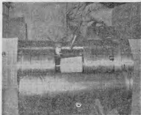
VASO INYECTADO EN CILINDRO CALIENTE. Esta máquina está en capacidad de producir doscientos vasos por hora. El producto es de un hermoso acabado y de muy alta calidad. El vaso plástico, del tipo irrompible, es mostrado aquí.
